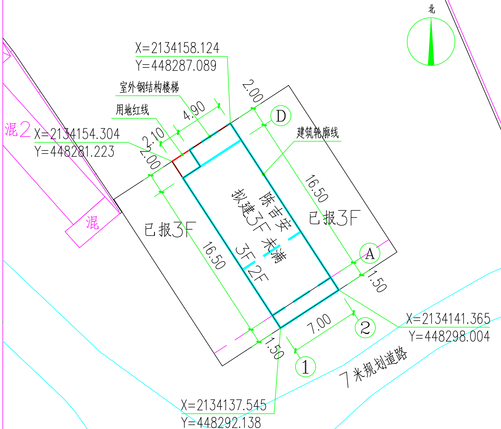
总 平 面 图
