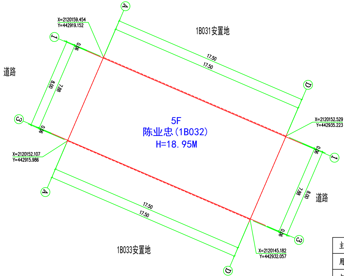
总平面图 1:100
